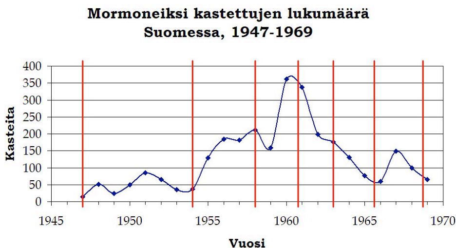
Kuva 2. Mormonilähetysohjön tuloksia Suomessa, 1947–1969.
