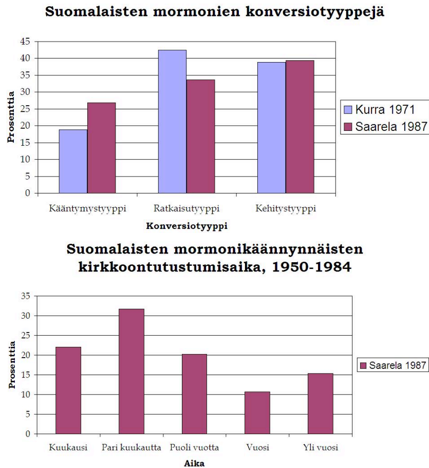
Kuva 1. Suomalaisten mormonikäännynnäisten (a) konversiotyyppijakaumia sekä (b) tutustumisajan pituus.
